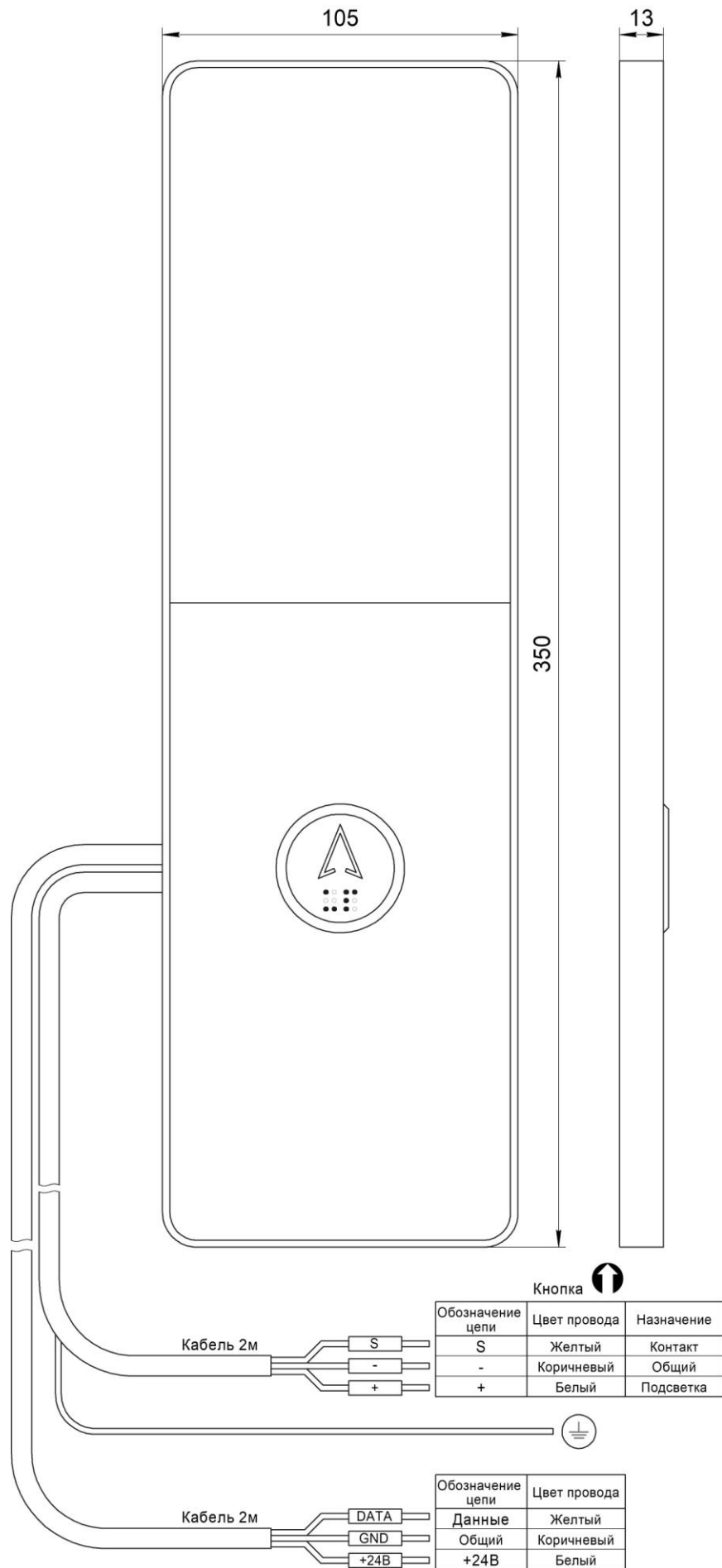
Рис.1 Внешний вид, габаритные и установочные размеры Вызывного поста МАЛАХИТ НШЕК.468381.025
